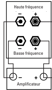
Connexions pour bi-câblage
