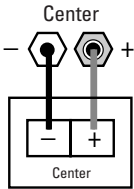
Sorties haut-parleurs de l'ampli-tuner
