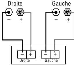
Sorties haut-parleurs de l'ampli-tuner
